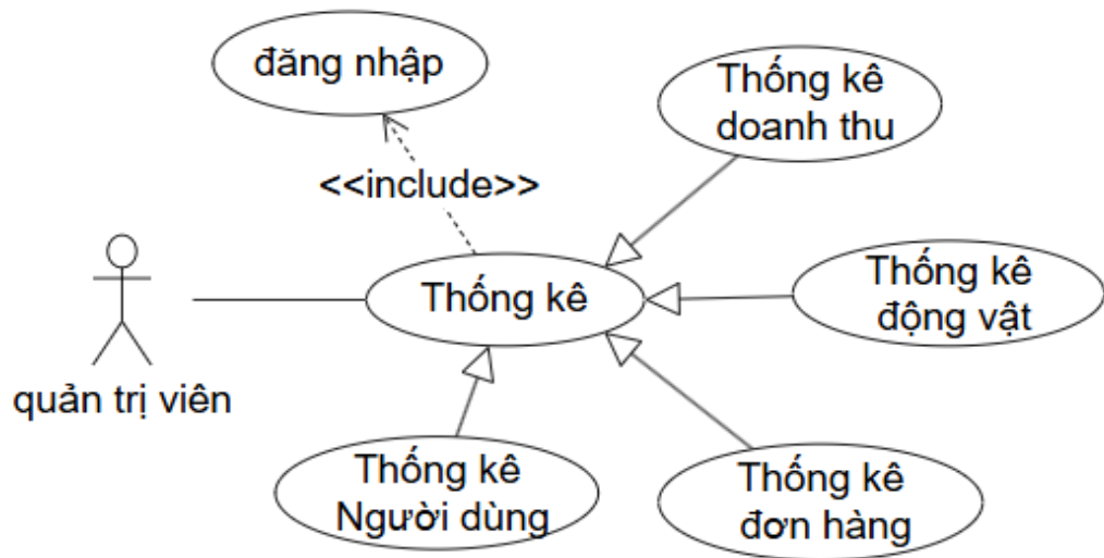
Hình 1.16 UseCase Thống kê
