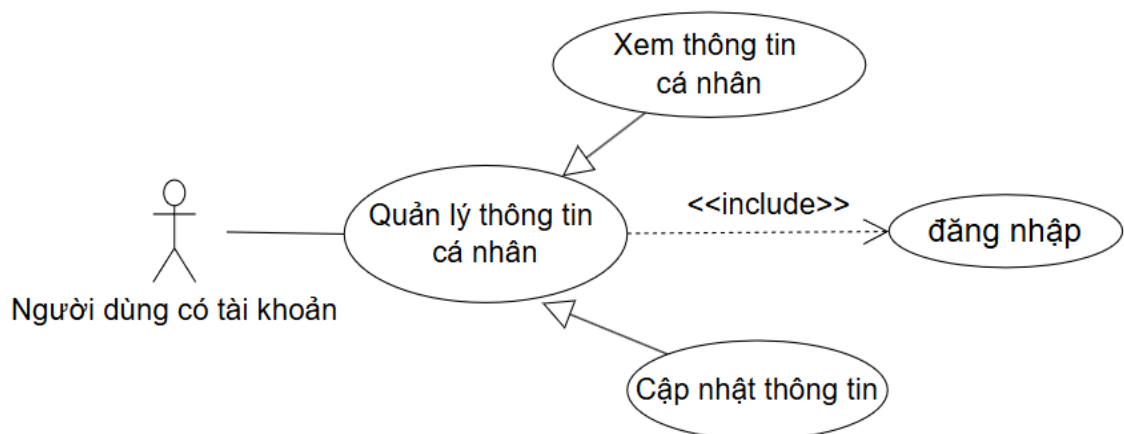
Hình 1.10 UseCase quản lý thông tin cá nhân
