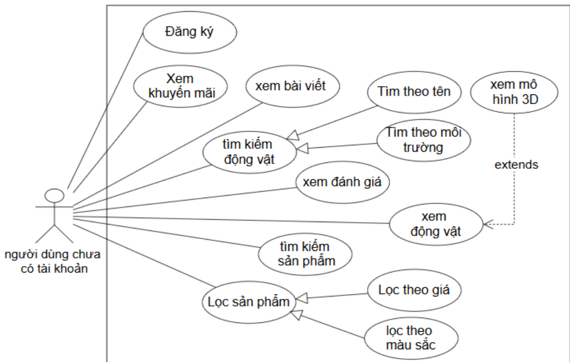
Hình 1.3 Sơ đồ UseCase tác nhân người dùng chưa có tài khoản
