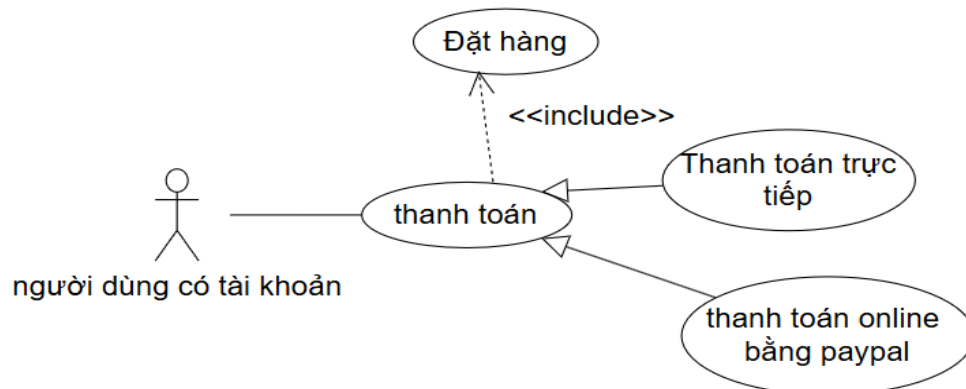
Hình 1.18 UseCase Thanh toán
