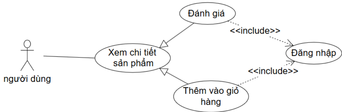
Hình 1.17 UseCase Xem chi tiết sản phẩm
