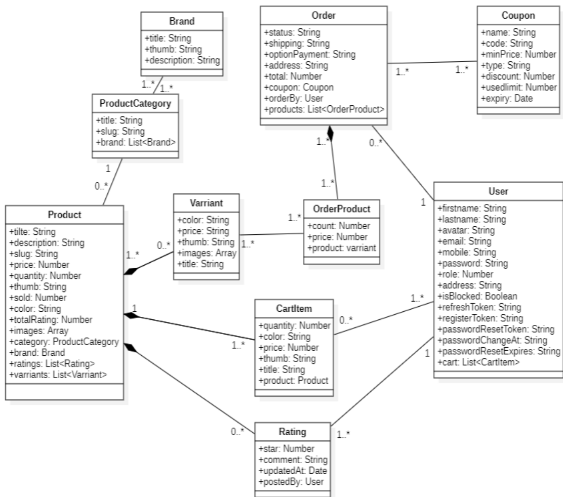
Hình 3.3 Sơ đồ lớp
