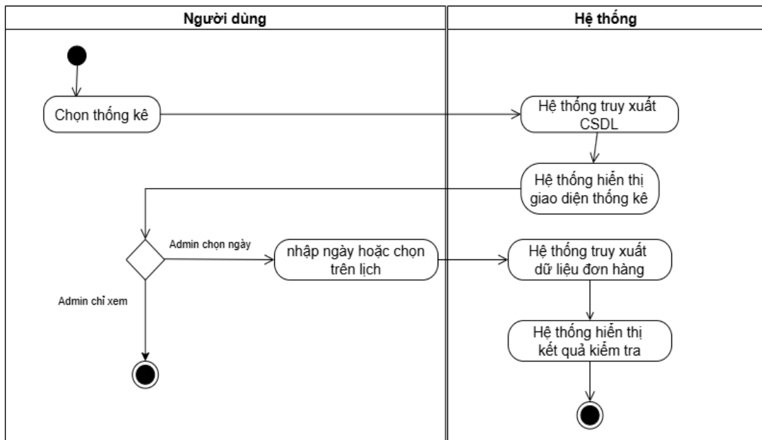
Hình 3.26 Sơ đồ hoạt động chức năng thống kê
