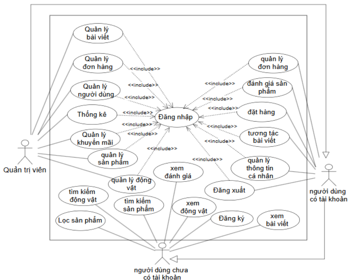
Hình 1.1 Sơ đồ UseCase tổng quát của các tác nhân
