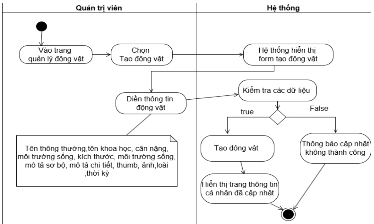
Hình 3.32 Sơ đồ hoạt động tạo động vật
