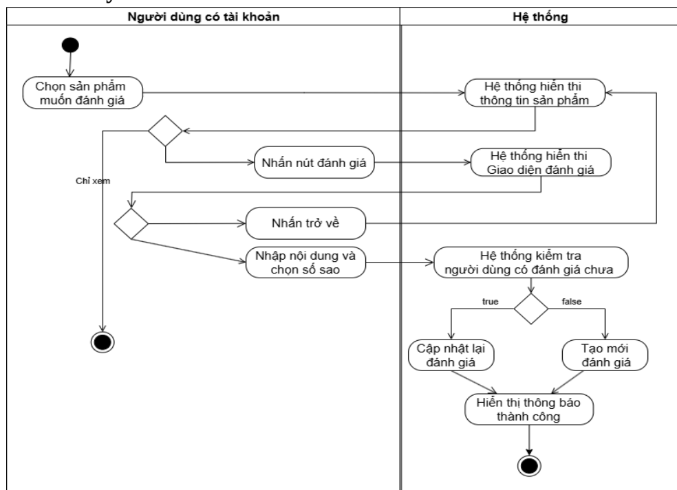
Hình 3.28 Sơ đồ hoạt động đánh giá sản phẩm
