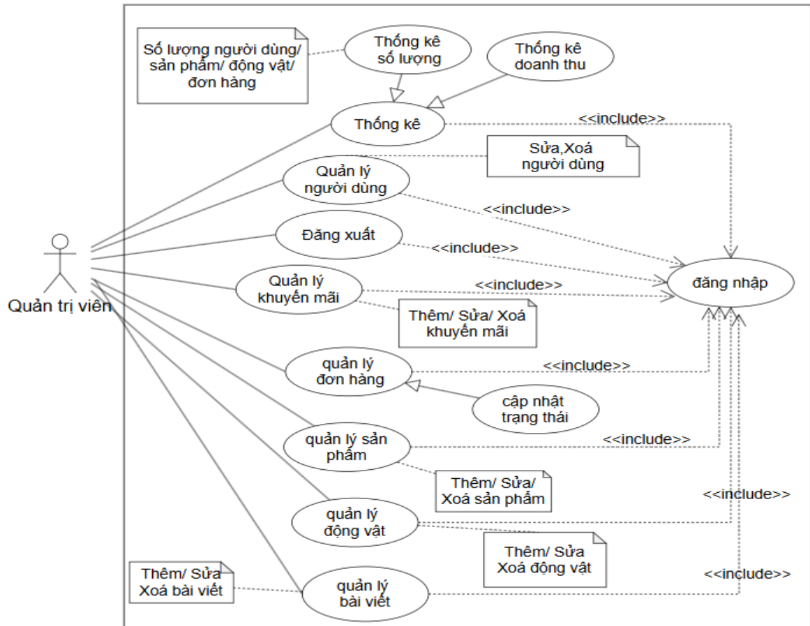
Hình 1.2 Sơ đồ UseCase của tác nhân Quản trị viên
