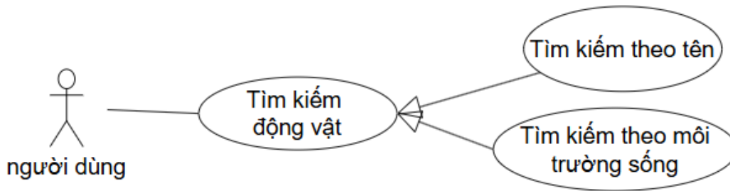
Hình 1.8 UseCase Tìm kiếm động vật
