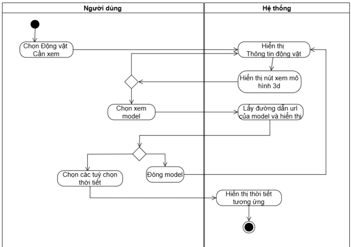
Hình 3.30 Sơ đồ hoạt động xem mô hình 3D
