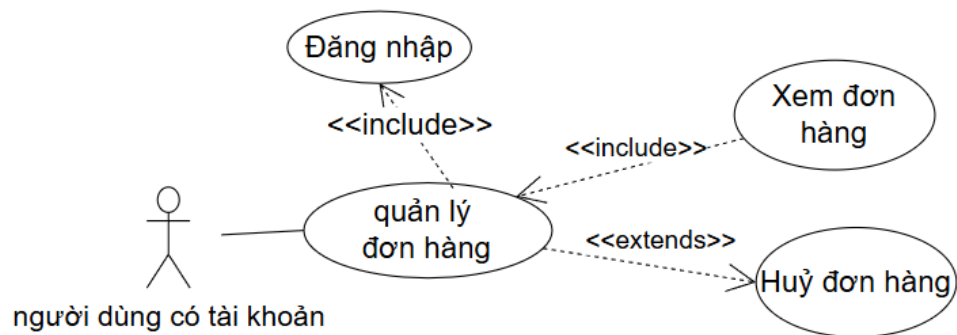
Hình 1.21 UseCase Quản lý đơn hàng(người dùng)
