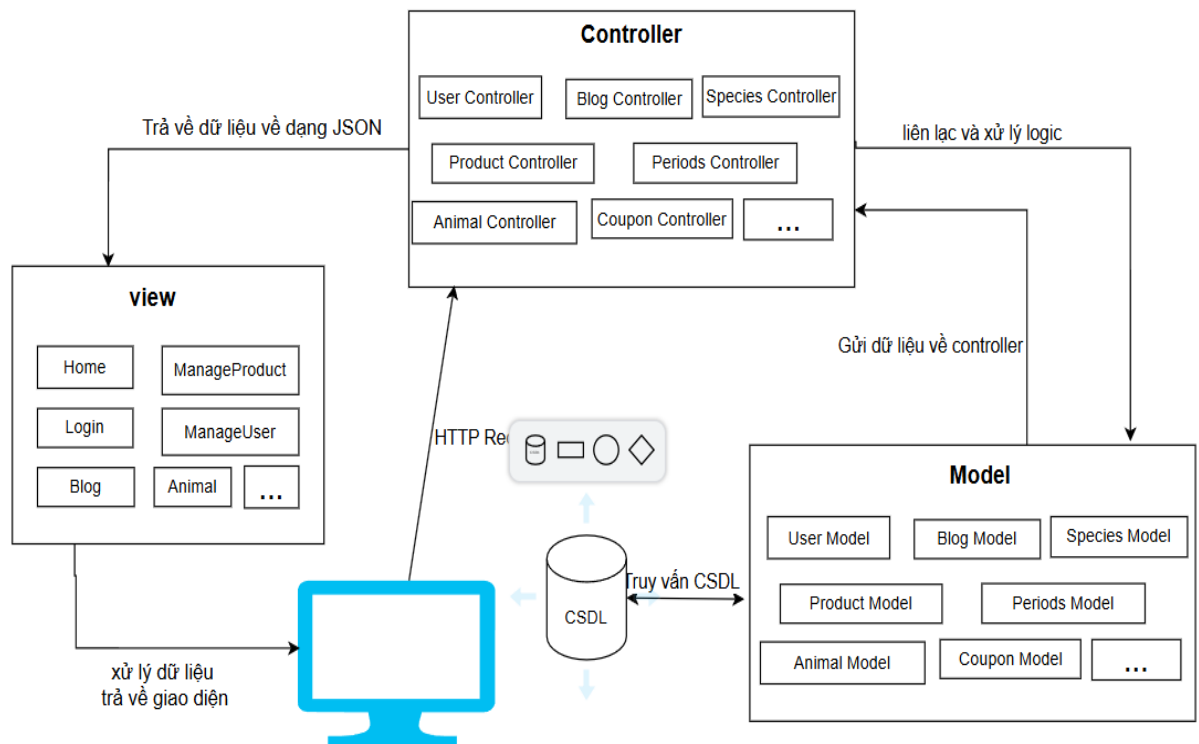
Hình 3.2 Mô hình MVC hoạt động
