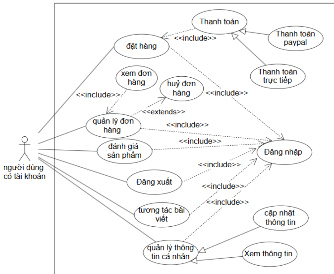
Hình 1.4 Sơ đồ UseCase của tác nhân Người dùng có tài khoản
