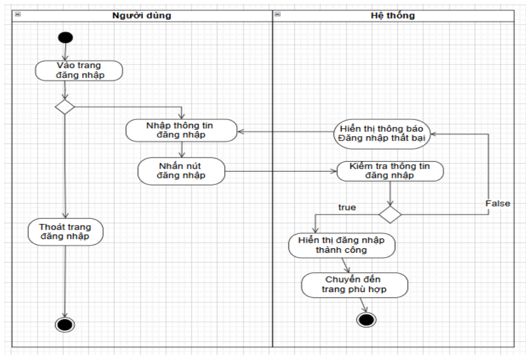
Hình 3.16 Sơ đồ hoạt động chức năng đăng nhập
