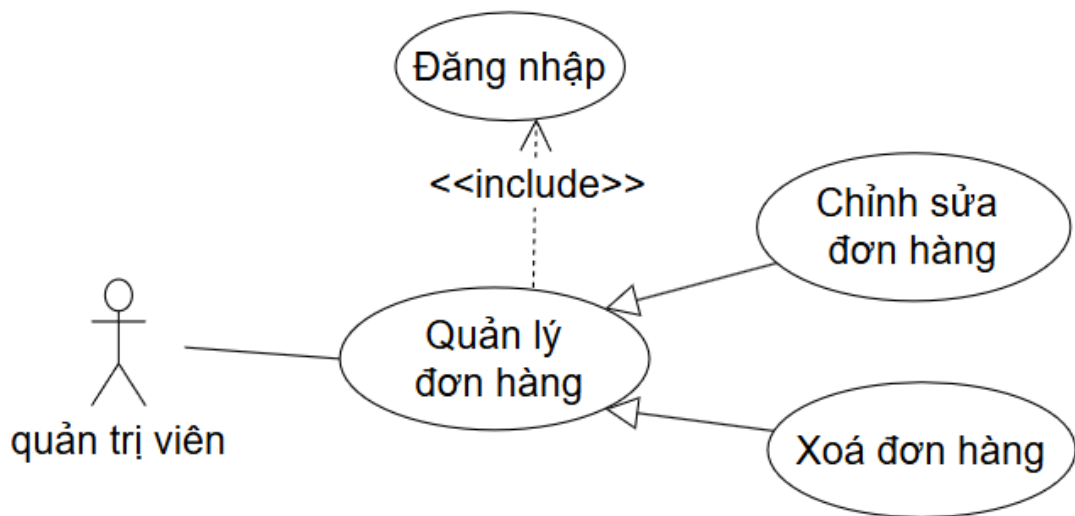
Hình 1.20 UseCase Quản lý đơn hàng
