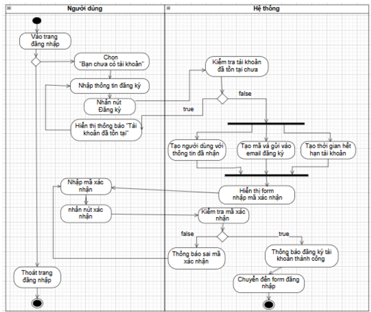
Hình 3.18 Sơ đồ hoạt động đăng ký
