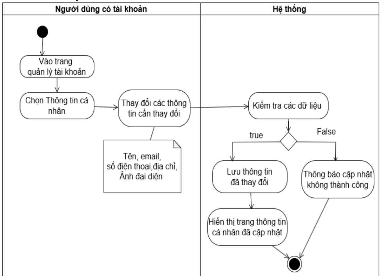
Hình 3.22 Sơ đồ hoạt động quản lý thông tin cá nhân
