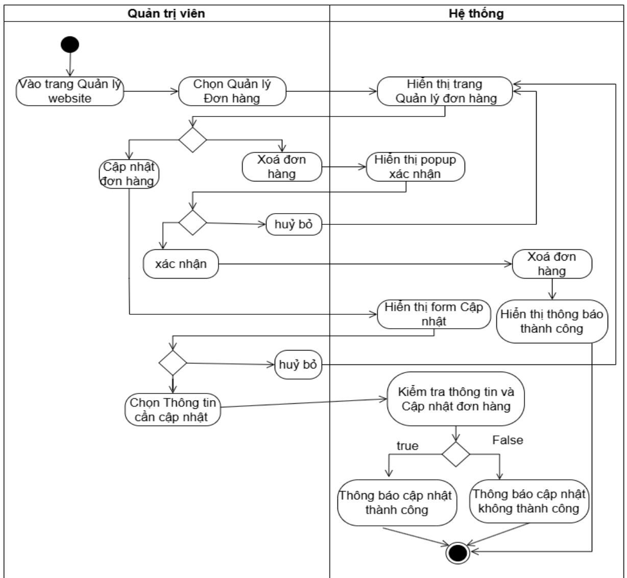
Hình 3.24 Sơ đồ hoạt động quản lý đơn hàng
