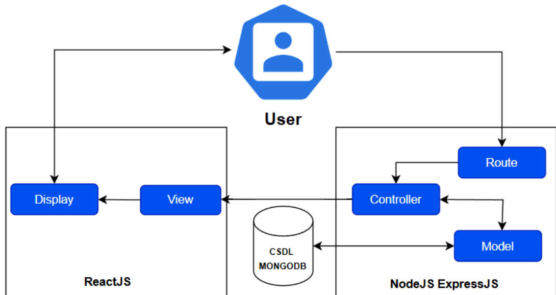
Hình 3.1 Mô hình hoạt động hệ thống
