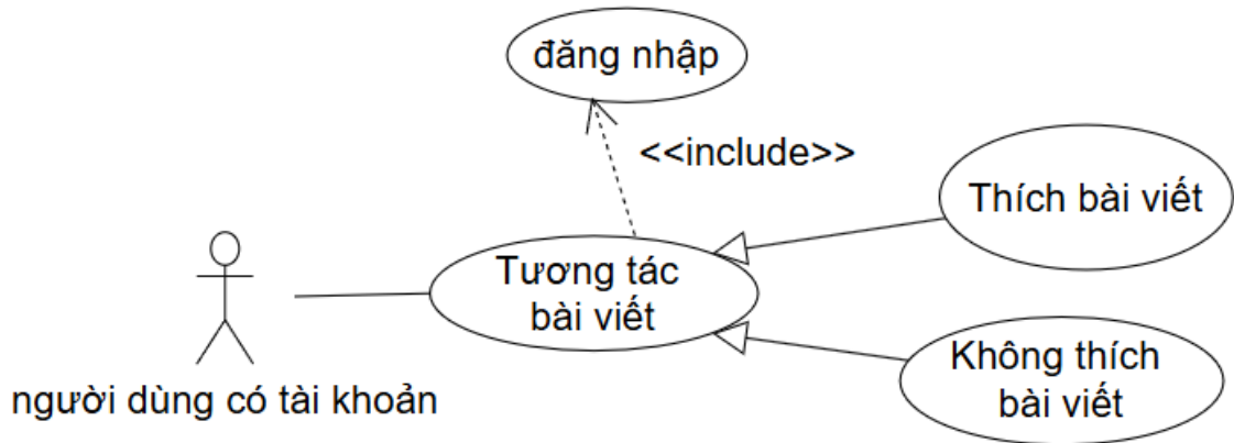
Hình 1.15 UseCase Tương tác bài viết
