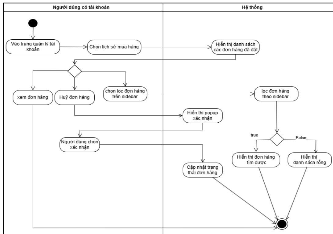
Hình 3.34 Sơ đồ hoạt động quản lý đơn hàng
