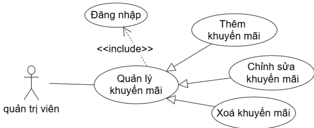
Hình 1.19 UseCase Quản lý khuyến mãi
